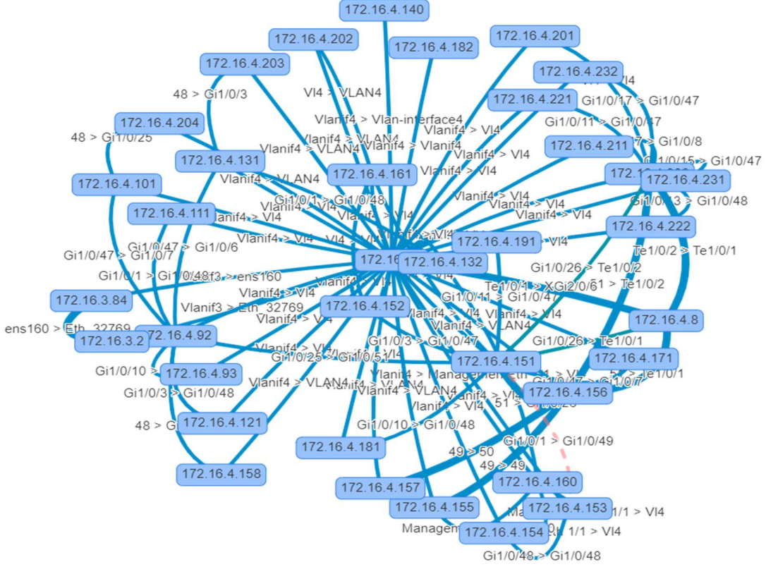
Şekil 1.1 Ağ Mimarisi
