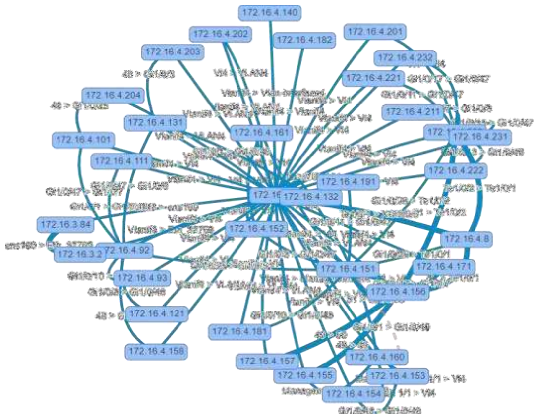
Şekil 1.1 Ağ Mimarisi
